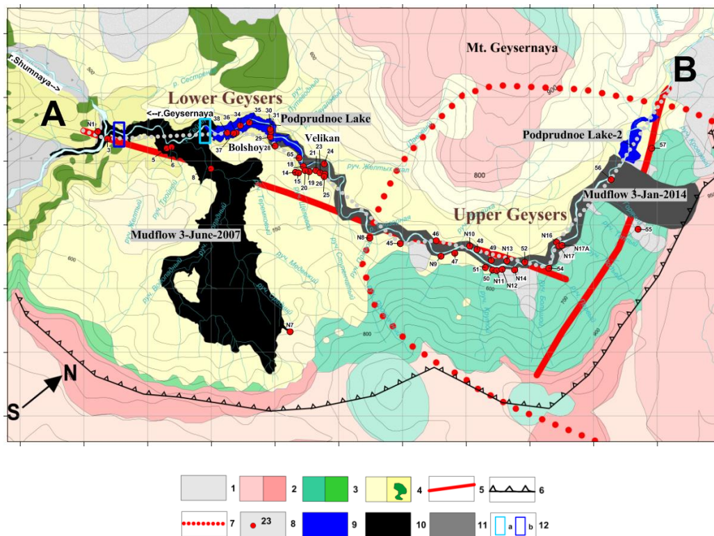
Рис. 4. Схематическая карта Долины Гейзеров. Легенда: 1 – аллювиальные и ледниковые отложения Q_{3-4} ; 2 – проницаемые блоки риолитовых, дацитовых и андезитовых экструзий ( \alpha Q_3^4 ); 3 – базальтовые, андезитовые, и дацитовые лавы и пирокластика ( \alpha Q_3^{1-2} ); 4 – блоки низко проницаемых кальдерно-озерных отложений ( Q_3^4 ), осложненные комплексом даек ( Q_3^{ust} ); 5 – предполагаемые термовыводящие разломы; 6 – граница Узон-Гейзерной депрессии; 7 – возвышенная область, связанная с предполагаемым контуром активного магматического резервуара (Lundgren et al., 2006); 8 – гейзеры и горячие источники (нумерацию см. в таблице 6 в работе Kiryukhin, 2016); 9 – Подпрудное озеро и Подпрудное озеро-2, сформированные оползнем и селем; 10 – катастрофический оползень-сель 3.06.2007; 11 – оползень-селевой поток 3.01.2014; 12 – точки измерения расхода реки Гейзерной: а – выход из Подпрудного озера, б – в устье р. Гейзерной. Размерная сетка – 500 м.
